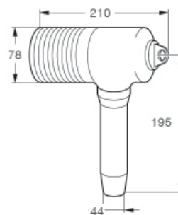
Elbow KAP 300 U.
